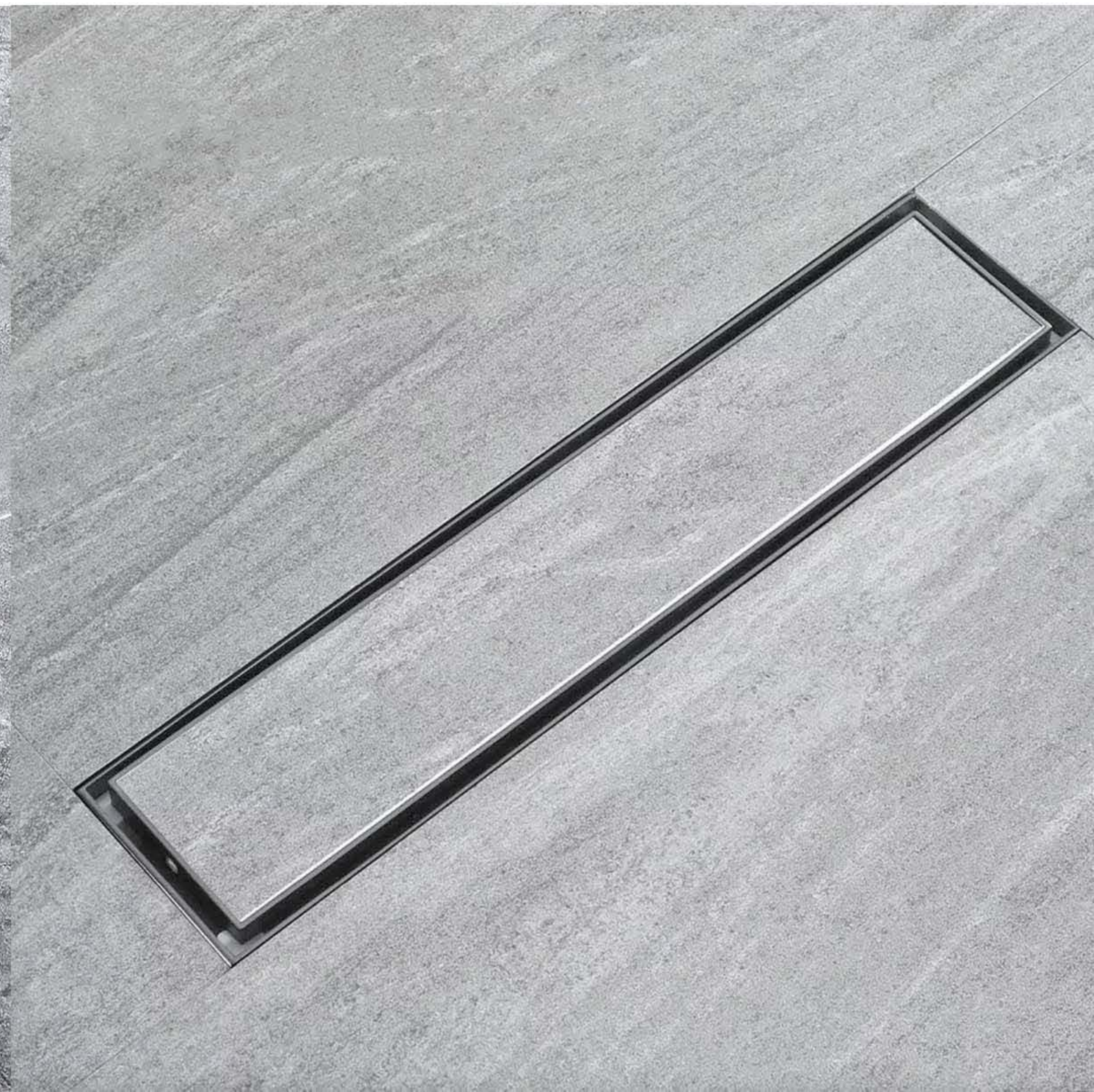
REJ-552 Rejilla rectangular invisible de 12" para empotrar en tubo de 2" REJ-502 Rejilla rectangular invisible de 24" para empotrar en tubo de 2" REJ-519 Rejilla rectangular invisible de 28" para empotrar en tubo de 2" REJ-532 Rejilla rectangular invisible de 32" para empotrar en tubo de 2" REJ-542 Rejilla rectangular invisible de 36" para empotrar en tubo de 2"
